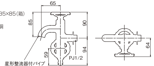
星形整流器付パイプ
