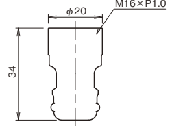
ワンタッチニップル(M16) G213WN ¥750 20/100
