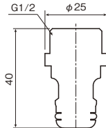
ワンタッチニップル外ネジ(メッキ) G203SN13M (限定在庫商品) ¥800 50/250
