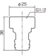
ワンタッチニップルの詳しい使い方をこちらのWeb動画から
