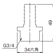
PPホースニップルセット 3C-3010 見積価格 1/50 ●材質:PP樹脂 ●UH・UP共用
