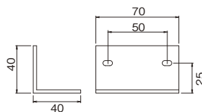
Rブラケット 3C-2900 見積価格 1/20 ●材質:Fe ●UH・UP共用
