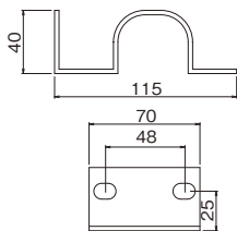
R3ブラケット 3C-2920 見積価格 1/20 ●材質:SUS304 ●UH・UP共用
