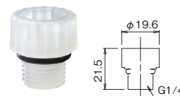
UPDレインプラグ (EPDM) 3C-S118000 見積価格 1/100 ●Oリング:EPDM
