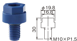
UHエアイベントプラグ (EPDM) 3C-S118021 見積価格 1/100 ●Oリング:EPDM
