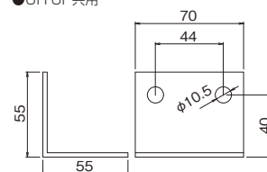
R2ブラケット 3C-2910 見積価格 1/20 ●材質:SUS304 ●UH・UP共用
