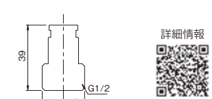
逆止弁セット G6-S ¥3,600(税込¥3,960) -/1 ●材質:黄銅 ●対応製品:KDS217-M
