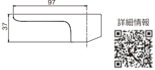
シングルレバーハンドル(ホワイト) LH-H-W ¥8,600(税込¥9,460) -/1 ●材質:亜鉛 ●対応製品:TK16NF-W, TK16NFP-W
