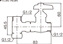
㊦ アンゲル分岐栓 AS13VK (受注生産品) ¥4,500 (税込¥4,950) 2/50
