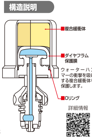
リリーフェース(水栓上部型) HV-201SPH ¥7,600(税込¥8,360) 1/50
