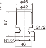
リリーフェース(止水栓補助型) HV-201CH ¥9,200(税込¥10,120) 1/50
