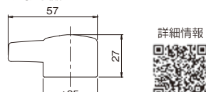
浄水吐水ハンドル SJ-KHM2 ¥2,000(税込¥2,200) -/1 ●材質:ABS樹脂 ●対応製品:KDS217-M
