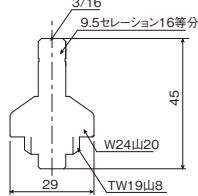
規格上部ハンドル無 KJ13-N ¥700(税込¥770) 1/100
