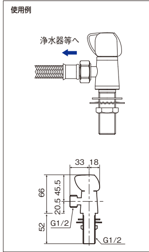
立形専用水栓 BP205TS-HH ¥7,000(税込¥7,700) 1/25
