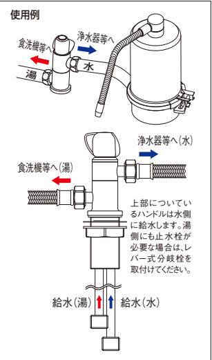
2方向分岐立形専用水栓(湯・水) BP205TSY ¥15,000(税込¥16,500) 1/10
