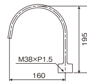
浄水器専用水栓パイプセット JF-PC 見積価格 -/1
