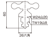
規格上部(クロスハンドル仙徳メッキ) KJ13-XMS ¥4,500(税込¥4,950) 10/100
