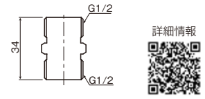
1/2ストレートニップル D-372-0 (受注生産品) ¥360(税込¥396) 50/600
