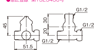
㊦ 片ナット付き分岐栓 (D式) AS207VK ¥4,200 (税込¥4,620) 1/50
