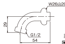
回転吐水パイプネジ付メッキ有 G205-NP ¥1,300(税込¥1,430) 10/100
