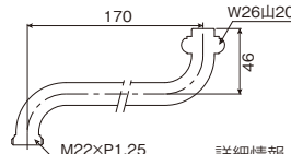
ねじ付自在パイプ170ミリ RP17N ¥1,600(税込¥1,760) 10/100
