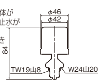
リリーフェース(水栓上部型) HV-201SPH ¥7,600(税込¥8,360) 1/50
