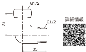
片ナットエルボ(研磨・メッキ付) JE204KT (受注生産品) ¥2,200(税込¥2,420) 20/120
