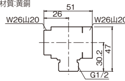
切替栓 BP12KS (既定在庫商品) 見積価格 10/50
