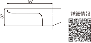
シングルレバーハンドル LH-H ¥4,600(税込¥5,060) -/1 ●材質:亜鉛 ●対応製品:TK16NFP, TK16NF
