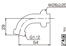
回転吐水パイプネジ付仙徳メッキ G205-MSP ¥3,000(税込¥3,300) 10/100
