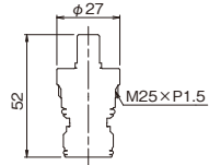
樹脂製セラミックカートリッジ JF-VJ ¥1,600(税込¥1,760) 10/100
