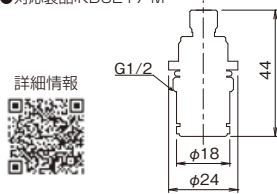
浄水吐水カートリッジ SC-GS ¥5,200(税込¥5,720) -/1 ●材質:黄銅・NBR ●対応製品:KDS217-M
