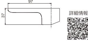
シングルレバーハンドル(ブラック) LH-H-B ¥8,600(税込¥9,460) -/1 ●材質:亜鉛 ●対応製品:TK16NF-B, TK16NFP-B
