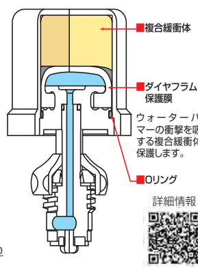
※ リリーフェース(水栓上部型) HV-201SPH
