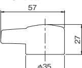
浄水吐水ハンドル SJ-KHM2 ¥2,000(税込¥2,200) -/1 ●材質:ABS樹脂 ●対応製品:KDS217-M
