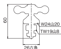
規格上部(クロスハンドル仙徳メッキ) KJ13-XMS ¥4,900(税込¥5,390) 10/100
