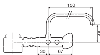
吐水口付シングルレバー分岐セット6×10 BP214TB-S6×10 見積価格 -/1
