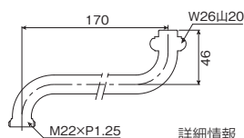
ねじ付自在パイプ170ミリ RP17N
