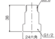
逆止弁3/8セット・AS G3-S ¥3,000(税込¥3,300) -/1 ●材質:黄銅 ●対応製品:TK216J
