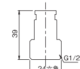
逆止弁セット G6-S ¥3,600(税込¥3,960) -/1 ●材質:黄銅 ●対応製品:KDS217-M
