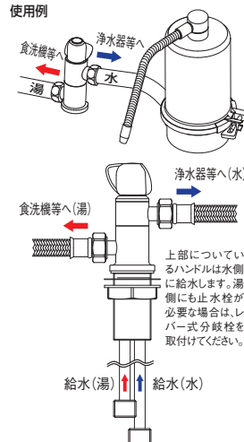
2方向分岐立形専用水栓(湯・水) BP205TSY
