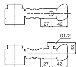
レバー式分岐付シングルレバー分岐セット6×10 BP205LB-S6×10 見積価格 -/1
