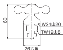
規格上部(クロスハンドルメッキ) KJ13-XM ¥2,800(税込¥3,080) 10/100
