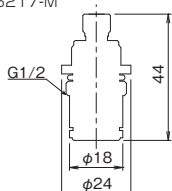
浄水吐水カートリッジ SC-GS ¥6,000(税込¥6,600) -/1 ●材質:黄銅・NBR ●対応製品:KDS217-M
