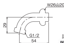
回転吐水パイプネジ付メッキ有 G205-NP
