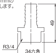
PPホースニップルセット 3C-3010 見積価格 1/50 ●材質:PP樹脂 ●UH・UP共用 ●内径12~15mmのホースに対応します。
