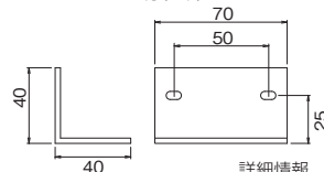
Rブラケット 3C-2900 見積価格 1/20 ●材質:Fe ●UH・UP共用 ●ボルト・ワッシャー付 (2本)
