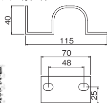
R3ブラケット 3C-2920 見積価格 1/20 ●材質:SUS304 ●UH・UP共用 ●ボルト・ワッシャー付 (4本)
