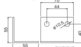
R2ブラケット 3C-2910 見積価格 1/20 ●材質:SUS304 ●UH・UP共用 ●ボルト・ワッシャー付 (2本)
