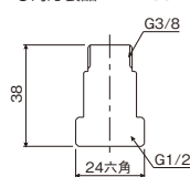
逆止弁3/8セット・AS G3-S ¥3,000(税込¥3,300) -/1 ●材質:黄銅 ●対応製品:TK216J
