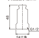
逆止弁セット G7-S ¥4,000(税込¥4,400) -/1 ●材質:黄銅 ●対応製品:手洗混合水栓161型シリーズ、手洗混合水栓162型シリーズ、手洗混合水栓コロレシリーズ
