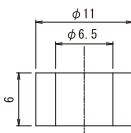
25用Bパッキン20個入り TK-B1 ¥2,000(税込¥2,200) -/1 重 量:0.1g ●材質:NBR
