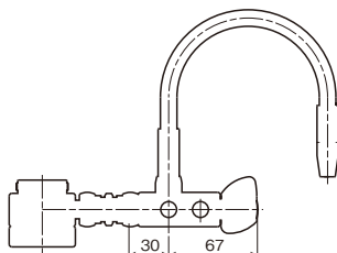
フレキ吐水口付シングルレバー分岐セット6×10 BP214FB-S6×10 見積価格 -/1
