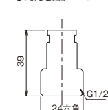
逆止弁セット G6-S ¥3,600(税込¥3,960) -/1 ●材質:黄銅 ●対応製品:KDS217-M
