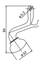
レバーハンドル湯用(赤) TKN-02R ¥3,000(税込¥3,300) -/1 重 量:80g ●材質:黄銅・ABS樹脂
