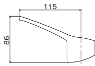
シングルレバーハンドル LH-E ¥4,600(税込¥5,060) -/1 ●材質:亜鉛 ●対応製品:KDS217-M
