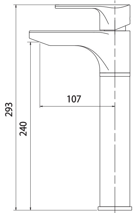
寸法図 [mm]
