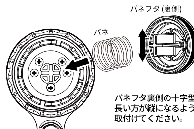
バネフタ (裏側)
